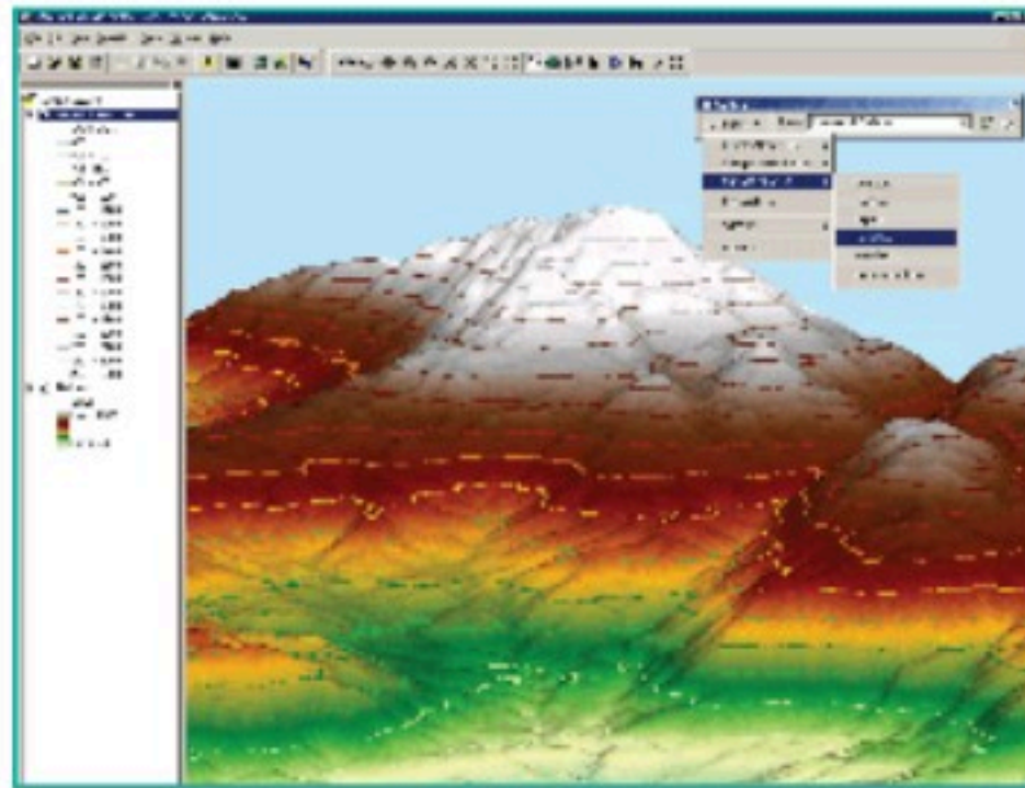
برنامج ArcGIS
