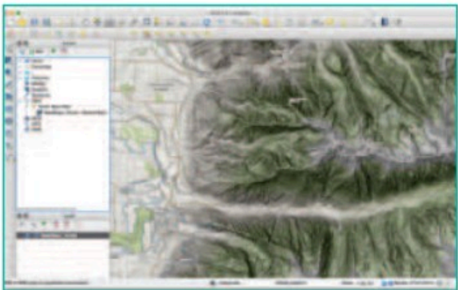
برنامج QGIS
